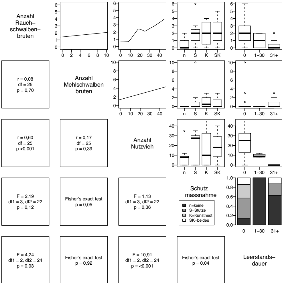
Abb. 1. Paarweise Korrelationen zwischen Anzahl Rauch- und Mehlschwalbenpaaren sowie Anzahl Nutzvieh, Leerstandsdauer und Art der Nisthilfen. In der oberen rechten Hälfte der Abbildung sind die Messdaten grafisch dargestellt, in der unteren linken Hälfte ist jeweils das Ergebnis des zugehörigen statistischen Tests angegeben. – Pair-wise correlation between numbers of Barn Swallow («Anzahl Rauchschwalbenbruten») and House Martin breeding pairs («Anzahl Mehlschwalbenbruten»), and the number of livestock («Anzahl Nutzvieh»), the type of artificial nest («Schutzmassnahme») and the duration of livestock absence («Leerstandsdauer»). In the upper right panel, the pair-wise relationships are presented graphically and in the lower left panel the corresponding statistical test results are given.
