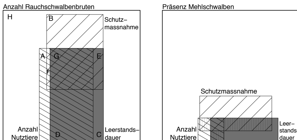
Abb. 2. Anteile der durch die drei Variablen «Nutztierzahl», «Leerstandsdauer» und «Nisthilfen» erklärten Devianz in der Anzahl Brutpaare von Rauchschnalben (links) und in der Präsenz von Mehlschnalben (rechts). Die Fläche des ganzen Rechteckes entspricht 100 % der Devianz in der Anzahl Rauchschnalbenpaare resp. in der Präsenz von Mehlschnalben. Die weisse, unschraffierte Fläche (H) entspricht dem Devianzanteil, der durch keine der 3 Variablen erklärt werden kann. Die Flächenanteile, die durch die drei schraffierten oder grauen Rechtecke markiert sind, entsprechen den durch die jeweilige Variable erklärten Devianzanteilen (s. Anhang). Überlappungen kommen durch Korrelationen unter den Variablen zustande. Punktiert schraffierte Flächen sind «negative» Überlappungen. Dies bedeutet, dass die erklärte Devianz im Modell mit beiden Variablen (um den punktiert schraffierten Flächenanteil) grösser ist als die Summe der erklärten Devianzen der beiden Modelle mit nur einer Variablen. – Proportions of explained variances in the number of Barn Swallow breeding pairs (left) and in the presence of House Martin (right). The total area corresponds to 100 % of the variance in the number of Barn Swallow breeding pairs and the presence of House Martin, respectively. The white, non-hatched area (H) is the proportion of variance that cannot be explained by any of the three predictor variables. The proportions of variance explained by each of the three predictor variables are given in hatched and grey rectangulars (see Appendix). There is overlap due to correlation between the variables. Dotted hatched areas are negative overlaps. This is, because the explained variance of the model including both predictor variables is larger than the sum of the explained variances of the two models containing each of the variables alone.
